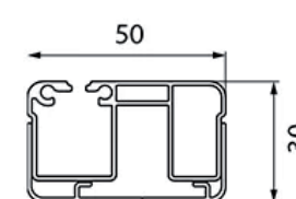
Profil coulisse moustiquaire manuelle
