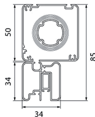
Profil coffre et barre de charge
