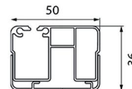
Profil coulisse moustiquaire motorisée
