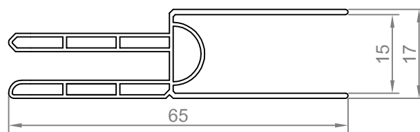
BATTEMENT PVC
