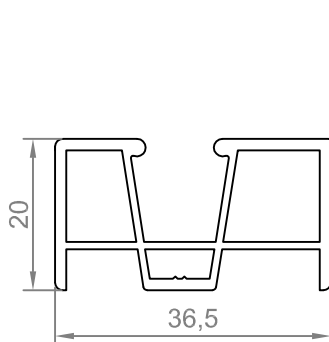
MONTANT PVC
